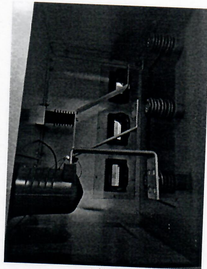
母排室
