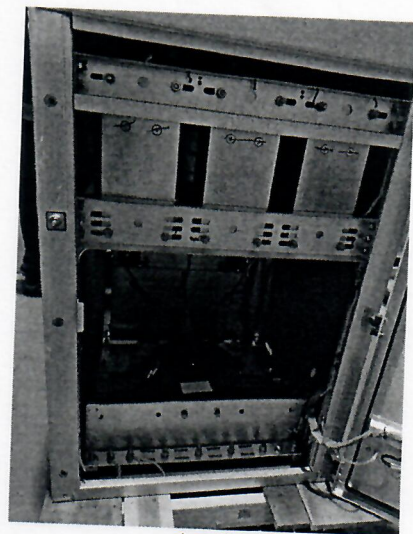
后下室
