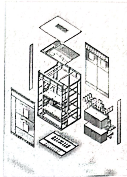
控制柜
