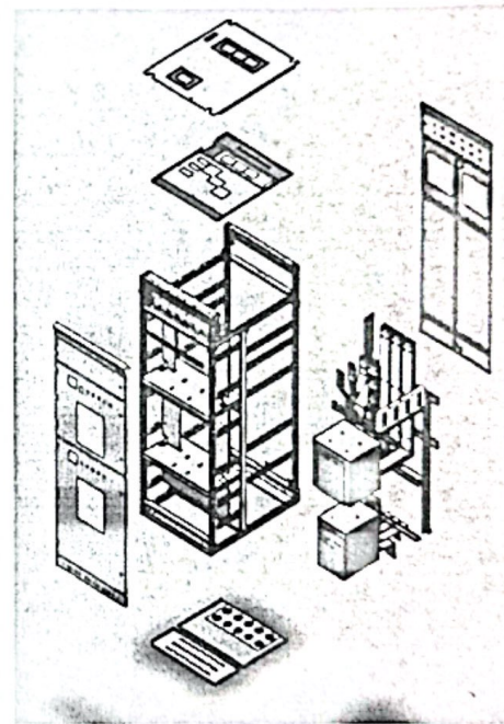
馈电柜
