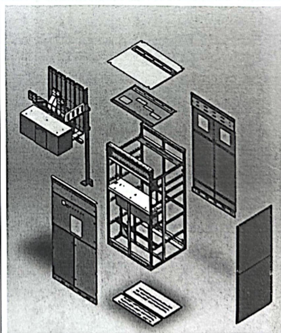
进线柜
